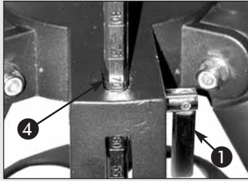
Fig. 47: Set latitude.
